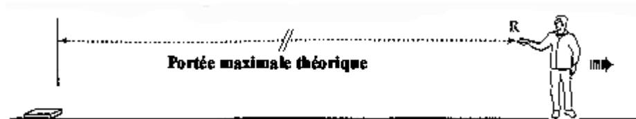
(Fig. 2) ARVA en émission au sol
